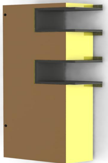
Рис. 7.2.1 Адаптация воздуховодов в вертикальной стенке кондиционируемого помещения (поз. 4 из комплекта поставки).
