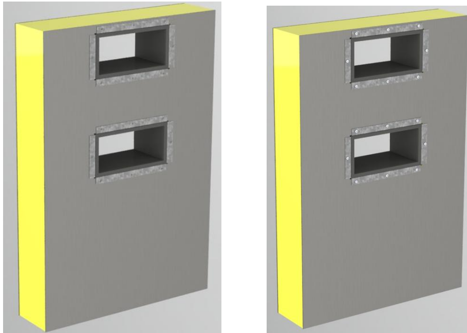
Рис. 7.2.2 Разметка отверстий и крепление воздуховодов.
