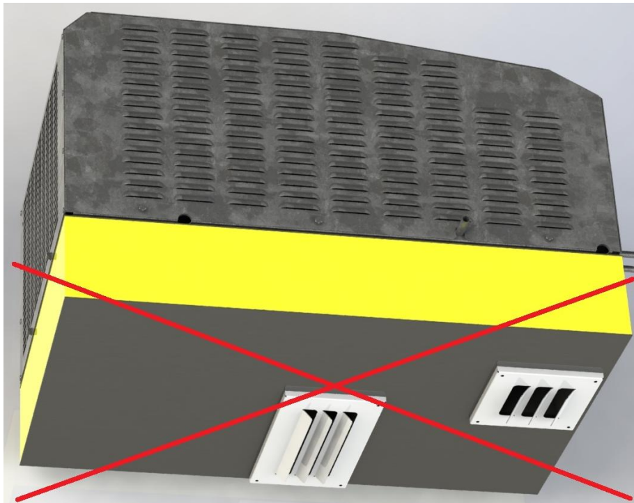
Рис. 7.4.2 Неправильное расположение решеток относительно друг друга.
