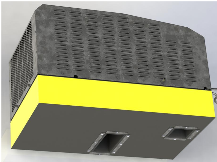
Рис. 7.3.2 Расположение кондиционера с установленными воздуховодами.
