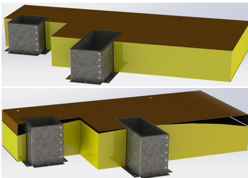
Рис. 7.2.1 Адаптация воздуховодов в крыше кондиционируемого помещения (поз. 6 и 7 из комплекта поставки).
