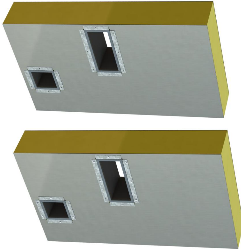
Рис. 7.2.2 Разметка отверстий и крепление воздуховодов.
