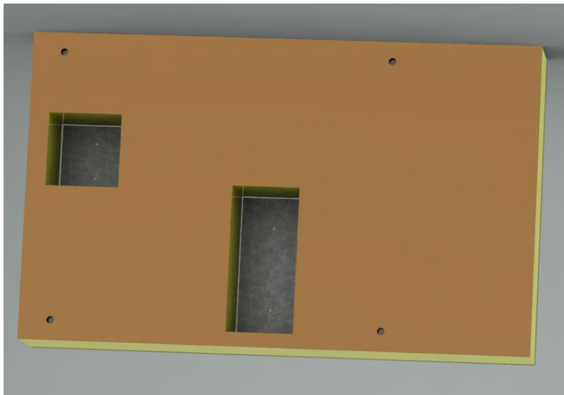
Рис. 7.1.3 Расположение шаблонов (поз. 3 и 4 из комплекта поставки) на внутренней стенке крыши с уличной стороны кондиционируемого помещения.
